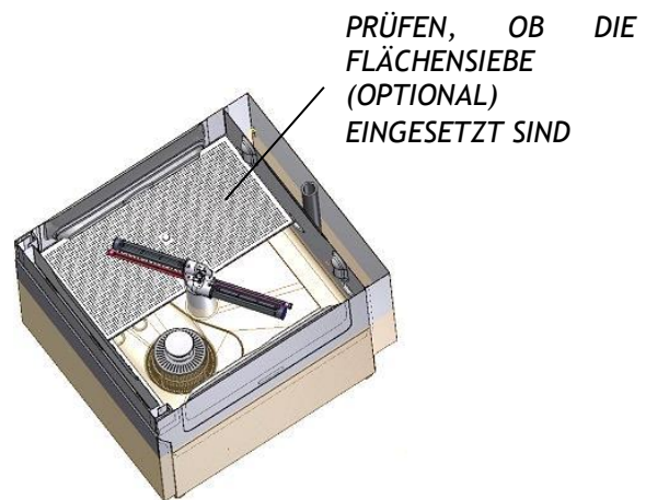
Innenansicht Tank
